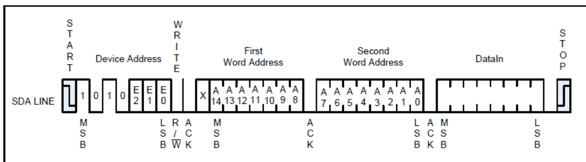
Figure8 : Byte Write
